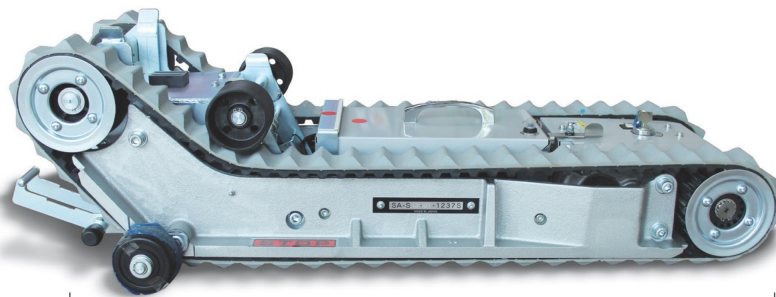
CZĘŚĆ JEZDNA
