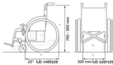
WÓZKI PASUJĄCE DO TRANSPORTERA (WYMIARY)
